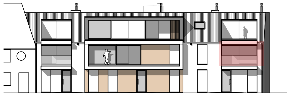
VOORGEVEL
